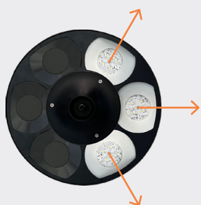
CD Led Evo composizione a 4 occhi CD Led Evo 4-eye configuration
