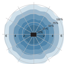
Curva fotometrica per installazione a soffitto Altezza di installazione consigliata: 2,5-6mt
