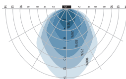
Curva fotometrica per installazione a parete Altezza di installazione consigliata: 1-1,8 mt
